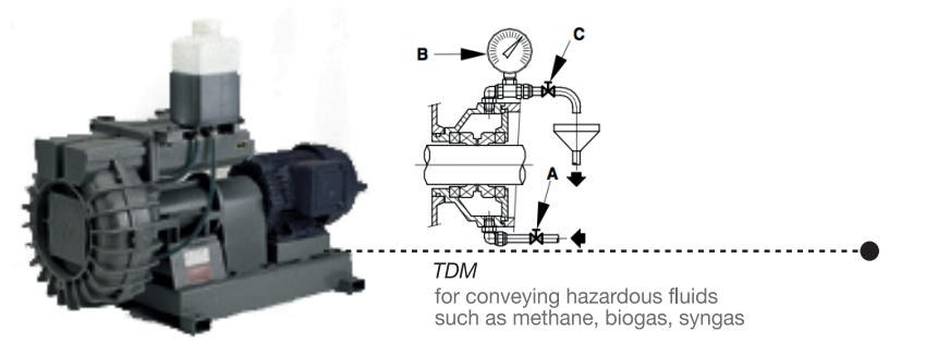
TS twin impeller single stage doppia girante singolo stadio doble impulsor mono etapa
